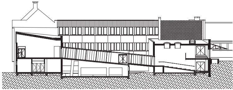
LANGSE SNEDE DOOR CORRIDOR
