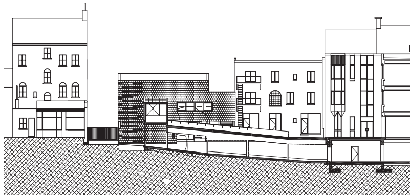
SNEDE 2 DOOR SPEELPLAATS
